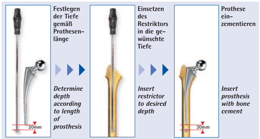
Applikator für Zementrestriktor Applicator for Cement Restrictor
